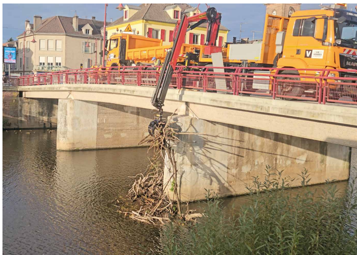
1 er octobre : les services du Département sont venus retirer les embâcles qui s'accumulaient dans la Meurthe au pied d'une pile du "pont de l'Union".
